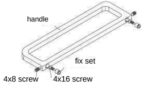
BNS-03 吊趟联动2+1(固定款)
