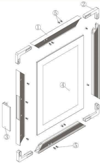
K3514 door frame
