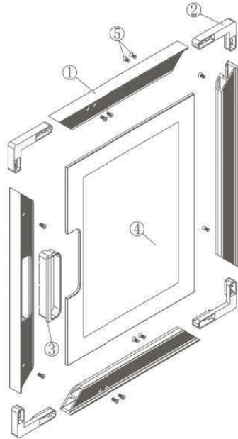
K3514 door frame
