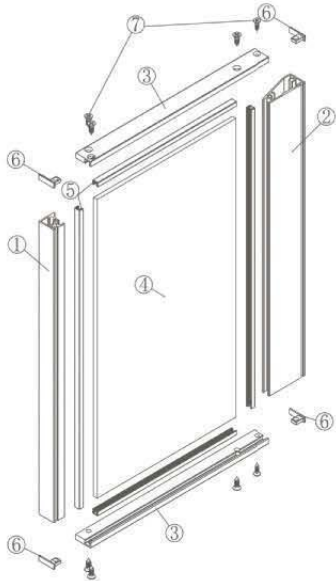
K3509 door frame
