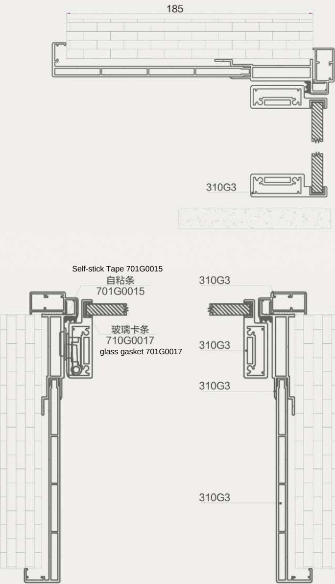
隐框平开门双包装配图(铝门套)
