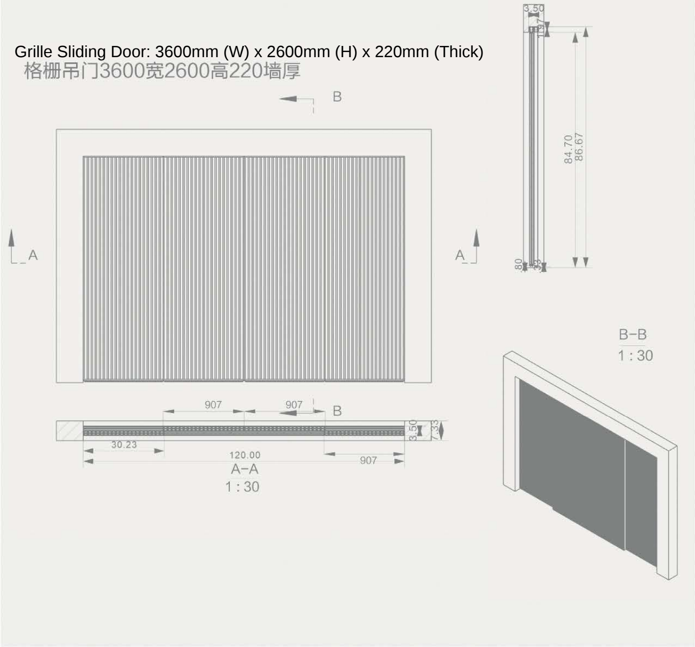
G3241 Grille Sliding Door Grille Slats G3241 格栅吊门格栅条
