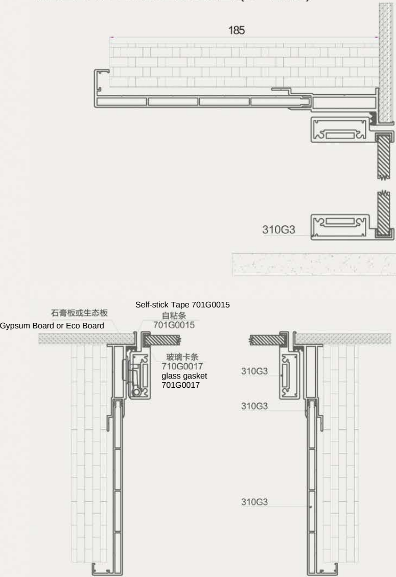
隐框平开门双包装配图(护墙板)
