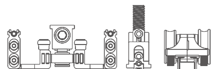
TN1098A 三联动中门滑轮配件套装
