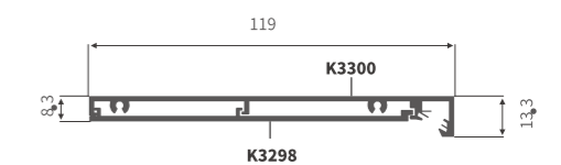
K3300/K3298 层板
