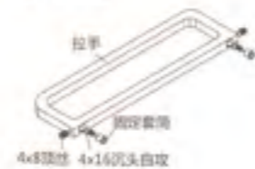
拉手(选配)
