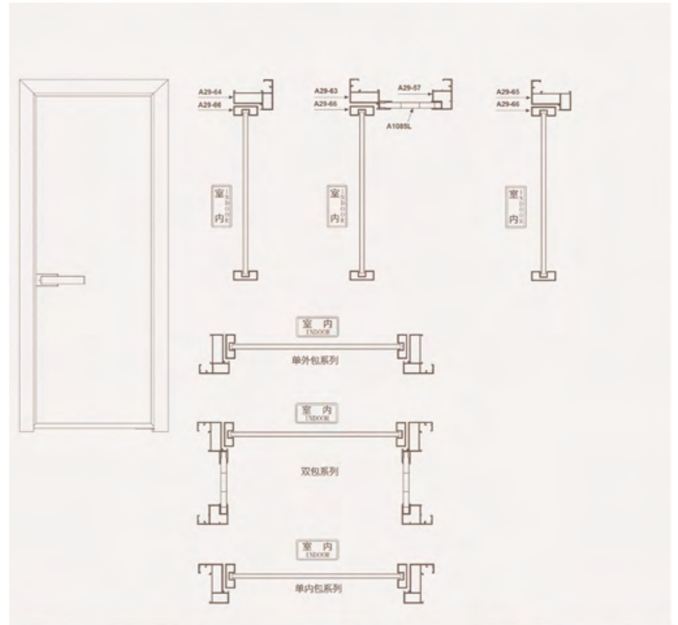
9-64 外包边框 A29-65 内包边框 A29-66 14天地 A29-57 双包外框
