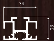
K3232 立柱
