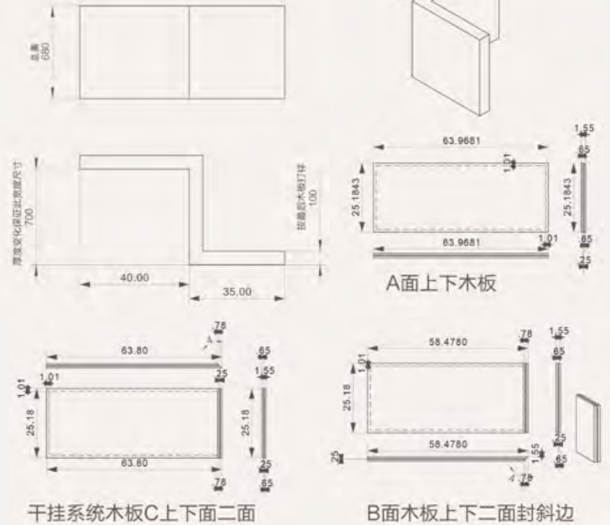
干挂式护墙 G3273 挂件 AC 下
