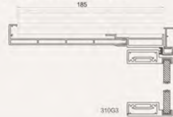
隐框平开门双包装配图(铝门套)
