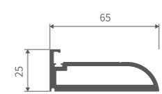
K2152 门框料
