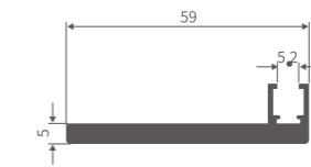
K3263 玻璃层板侧框
