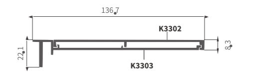
K3302/K3303 竖边板
