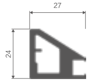
G3289 门框料
