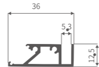
K2065 带灯槽框料
