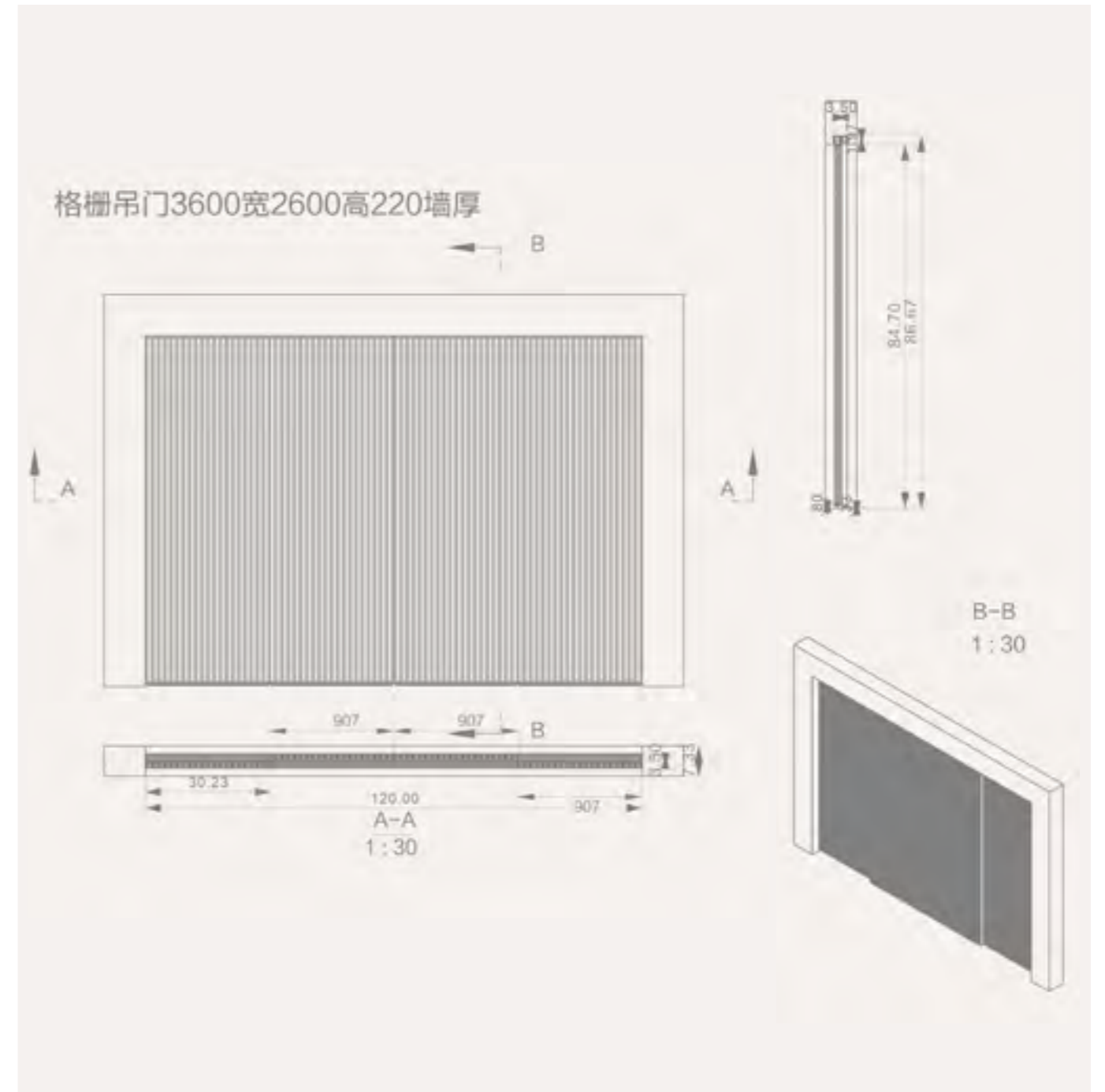
G3241 格栅吊门格栅条
