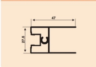
A-B8307 勾企 0.882kg/m
