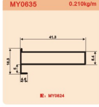
MY0635 0.210kg/m
