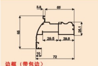
边框 (带包边)
