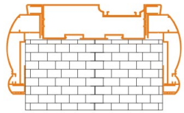
安装方式一
