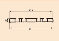
A-B8306 光企 0.804kg/m
