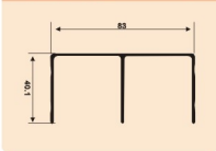
A-B8305P 下方 0.540kg/m
