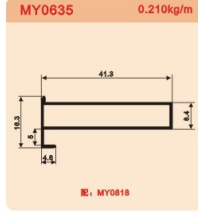
MY0635 0.210kg/m
