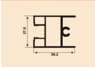
A-B8304P 上方 0.524kg/m
