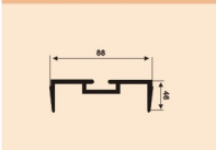
A-B8310P 光勾企盖板 0.145kg/m
