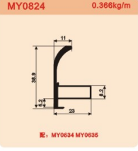
MY0824 0.366kg/m
