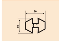
A-M5706 0.275kg/m
