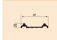
A-M5702 下轨 0.511kg/m
