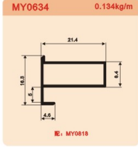
MY0634 0.134kg/m
