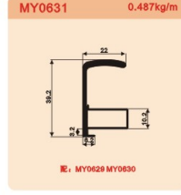
MY0631 0.487kg/m
