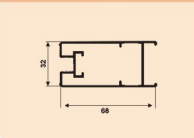
A-B8308P 中横 0.851kg/m
