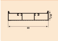
A-B8303P 边框 0.695kg/m
