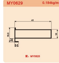
MY0629 0.184kg/m
