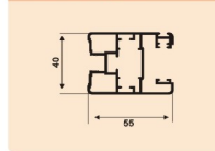
A-M5704T 平面光企 1.114kg/m
